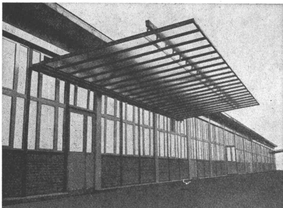
Glasvordächer in kittloser Konstruktion System WEMA
