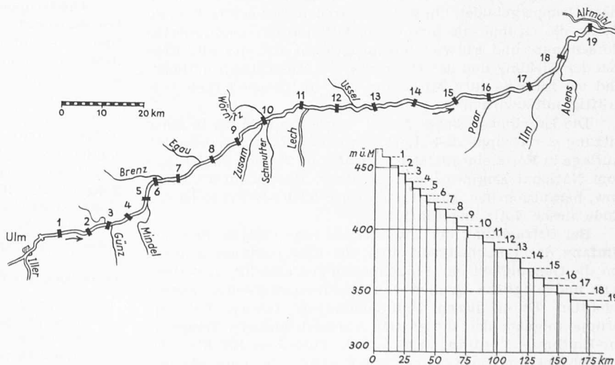
Bild 1. Donaustrecke Ulm-Kelheim, Uebersichtsplan 1:1,3 Mio und Längenprofil. Die Stufen heissen: 1 Oberelchingen, 2 Leipheim, 3 Günzburg, 4 Offingen, 5 Peterswörth, 6 Lauingen, 7 Dillingen, 8 Höchstädt, 9 Tapfheim, 10 Donauwörth, 11 Lechsend, 12 Bertholdshaus, 13 Bittenbrunn, 14 Bergheim, 15 Ingolstadt, 16 Grossmehring, 17 Wackerstein, 18 Eining, 19 Kelheim.
