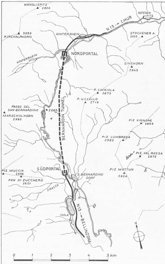
Bild 1. Bernhardintunnel, Lageplan 1:100 000
