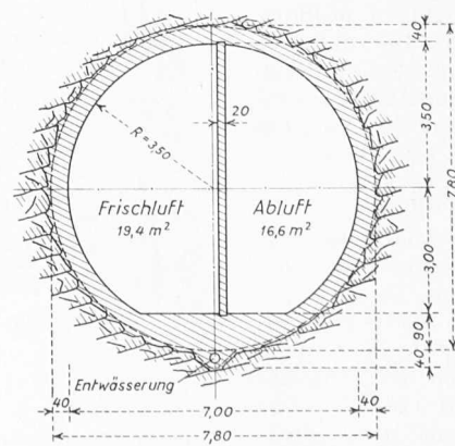
Bild 8. Lüftungs-Schrägschacht, Normalprofil 1:200
