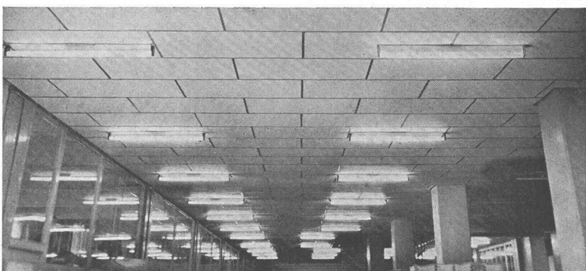
ungelochte Schallschluckplatte, unbrennbar, hier mit sichtbarem Hängerost in einem Druckereisaal
