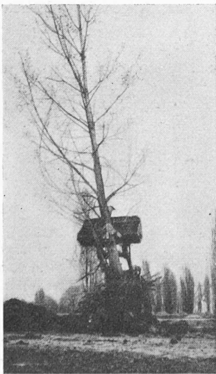
Verpflanzung grosser Bäume mit Hilfe eines dafür hergerichteten Schaufelladers
