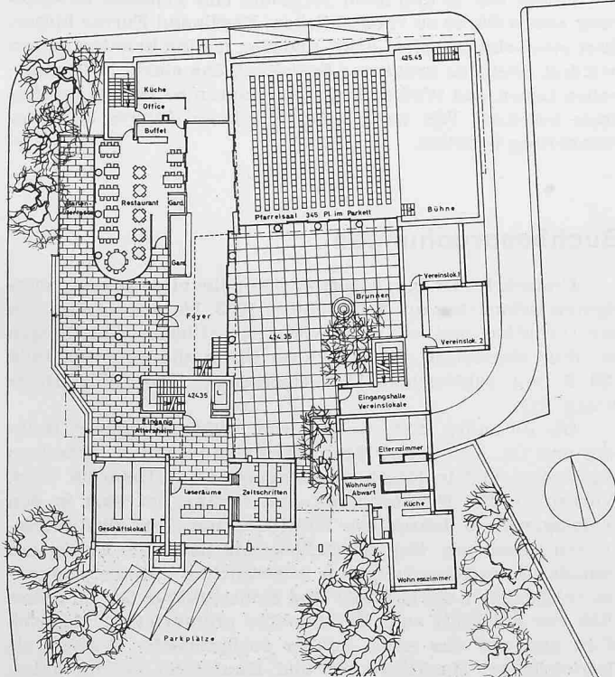
Erdgeschoss 1:600
