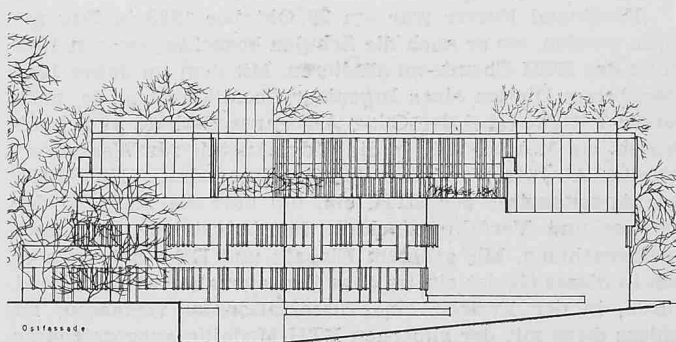
Ostfassade
