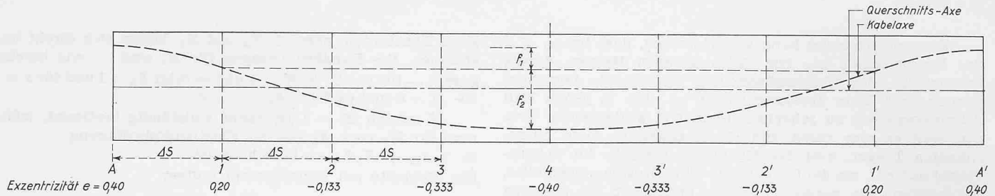
Bild 13. Trägerabwicklung. Längen 1:200, Höhen 1:50
