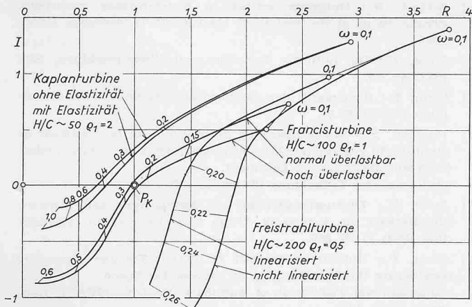
Bild 4. Reglereinstellung nach Optimum-Formel für Kaplan- und Francis-Turbinen. Ortskurven für den Frequenzgang F_0 des aufgeschnittenen Regelkreises zeigen durch den Verlauf gegenüber dem kritischen Punkt P_K der Stabilitätsgrenze den Einfluss der Elastizitätszahl \rho_1 (Größenordnung \sim 100 : H/C ). Für Kaplan- und Francis-Turbinen bis H/C \sim 50 ( \rho_1 = 2 ) ergeben die einfachen Optimum-Formeln eine weite Stabilitätsreserve durch grossen Abstand vom kritischen Punkt P_K . Bei H/C \sim 100 ( \rho_1 = 1 ) kommen Francis-Turbinen an die Stabilitätsgrenze. Bei H/C \sim 200 ( \rho_1 = 0,5 ) kommen bei der gleichen Reglereinstellung Freistrahlturbinen in das instabile Gebiet, besonders weit, wenn der Zusammenhang zwischen Wassermenge und Leistung nicht linearisiert ist.
