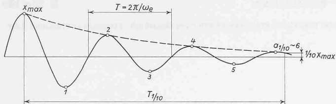
Bild 1. Als Kriterium für das Abklingen einer Störung auf 1/10 des maximalen Ausschlags x_{max} wird die Abklingzeit T_{1/10} eingeführt und die Anzahl Ausschläge a_{1/10} nach beiden Richtungen in dieser Zeit. a_{1/10} ist T_{1/10} : T/2 , wobei T die Zeitperiode 2\pi/\omega_e für eine ganze Regelschwingung ist.
