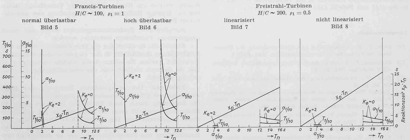
Bilder 5 bis 8. Kurven zur Auswahl der «besten» Reglereinstellung, unter Berücksichtigung konstruktiver Begrenzungen, durch Abwägen von Abklingzeit T_{1/10} , Anzahl a_{1/10} der Ausschläge und Reaktionszeit x_p T_n . Werte ohne und mit «künstlicher» Selbstregelung K_e > 0 mit Einführung einer Statik zwischen Frequenz und elektrischer Spannung. Durch Näherungsformeln (38) wird der Ausgangspunkt bestimmt. Die dargestellten Werte werden durch den Computer mit Iteration schnell vollautomatisch gerechnet, bei stufenweiser Eingabe für die Werte der Nachstellzeit (Isodromzeit) T_n . Beim hohen Wert der Selbstregelung K_e = 2 erreicht man bei kleinem T_n (Isodromzeit) praktisch aperiodischen Verlauf ( a_{1/10} \sim 0 ), kurze Abklingzeit T_{1/10} und schnelle Reaktion ( x_p T_n klein).
