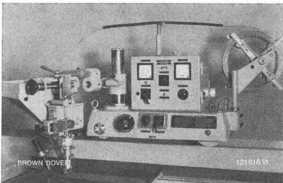
Universeller Lichtbogenschweissautomat für Gleich- oder Wechsel- stromschweissung, maximale Stromstärke 1200 A
