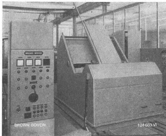
Mittelfrequenz-Induktions-Erwärmungsanlage mit Sägeautomat. Anlageleistung 100 kW, 4kHz; mittlerer Durchsatz ca. 400 kg/h.
