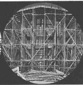
Lehrgerüst
