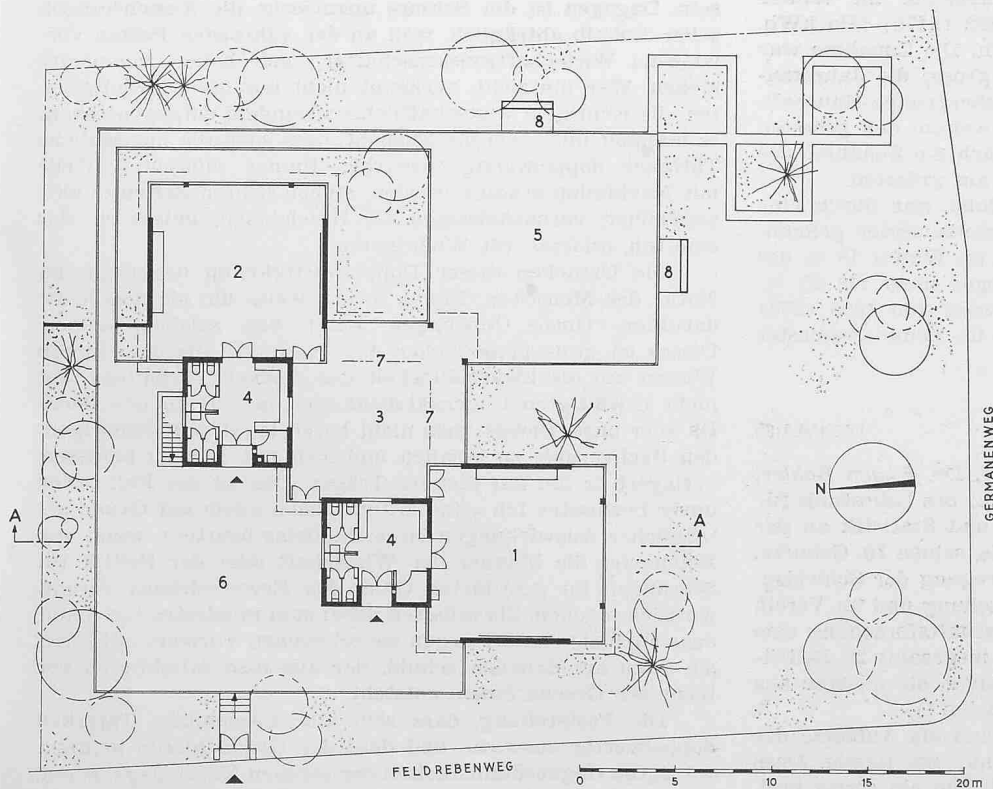
Grundriss 1:400
