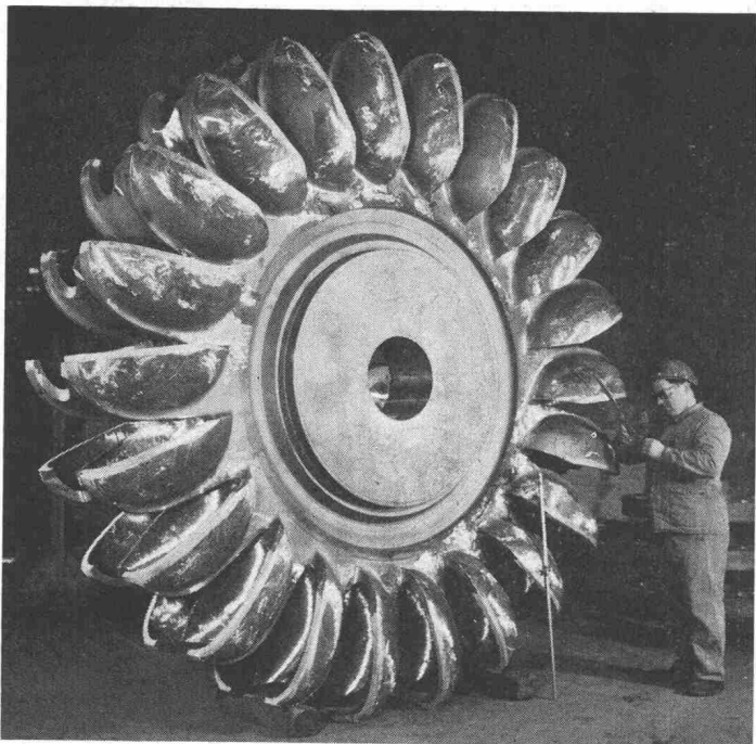
Bild 1. Ueber 10 t schweres, in einem Stück gegossenes Pelton-turbinenrad aus 13prozentigem Chromstahl
