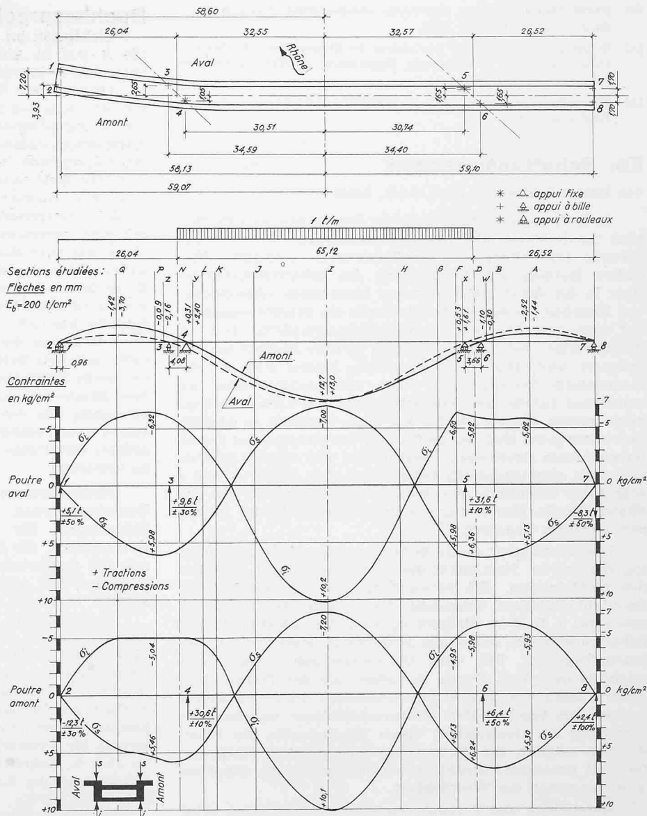
Diagramme de charge Flèches en mm Contraintes dans les deux poutres aval et amont sur les fibres supérieures \delta_s et inférieures \delta_i .
