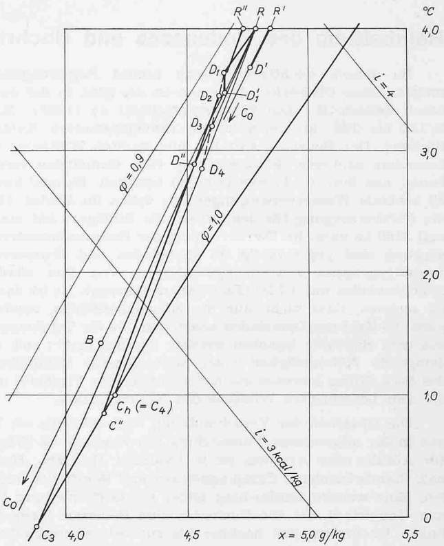
Bild 8. i , x -Diagramm mit den Zustandspunkten, die sich auf das im Text behandelte Beispiel beziehen. Die Punkte D 1 bis D 4 entsprechen dem Fall B bei den Aussen-temperaturen -10, 0, +10, +20 °C, die Punkte D' bzw. D'' dem Fall B 2 bei -10 bzw. +20 °C bei reinem Luftkühlerbetrieb jedoch erhöhter bzw. verringerter Raumfeuchtigkeit
