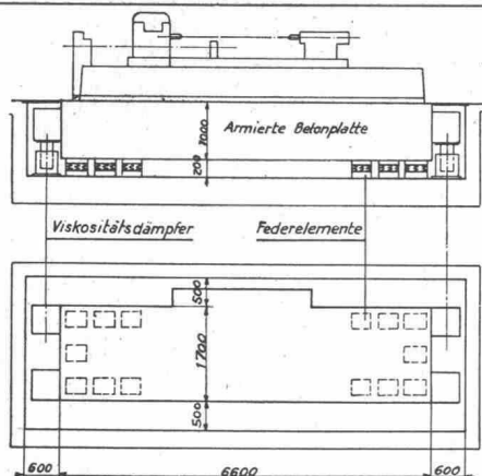
Schwingungsisol. Montage
