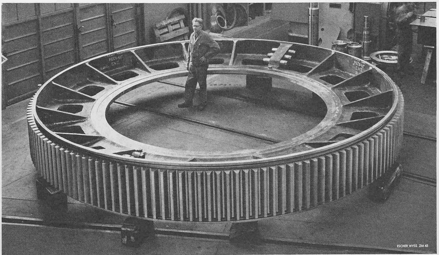
2. Zwillingantrieb
