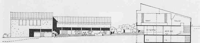
Schnitt Kirchgemeindehaus mit Ansichten Pfarrhaus und Kindergarten 1:700
