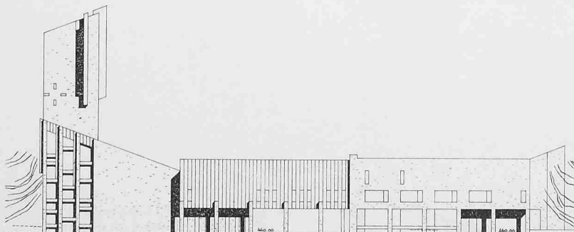
Südfassade 1:700
