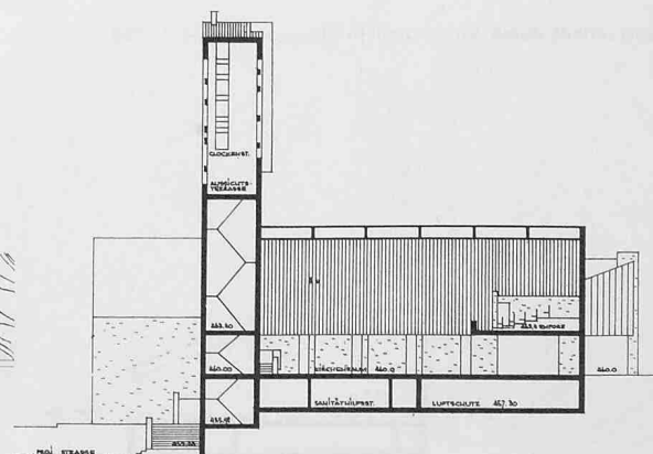
Längsschnitt durch Kirche 1:700
