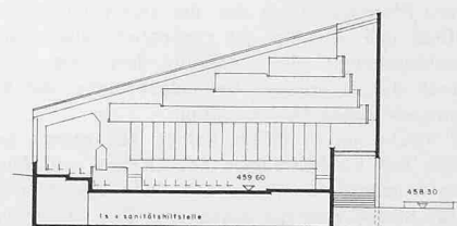
Schnitt Kirche 1:700
