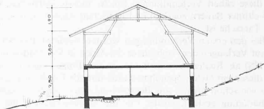
SNITT DURCH SCHEUNE
