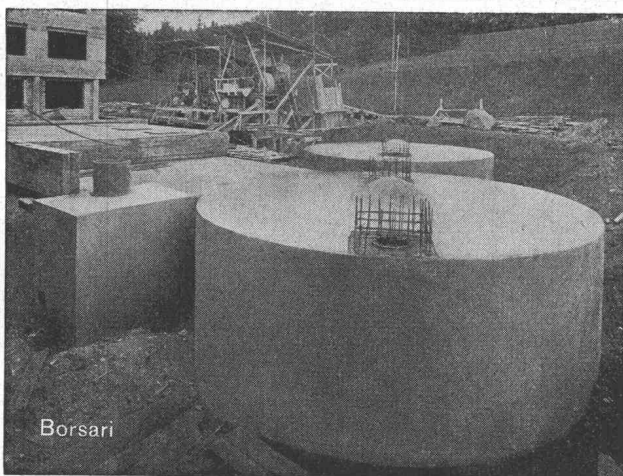
Altersheim Bethesda, Küsnacht ZH, 2 Tanks, total 400 m 3 Heizöl
