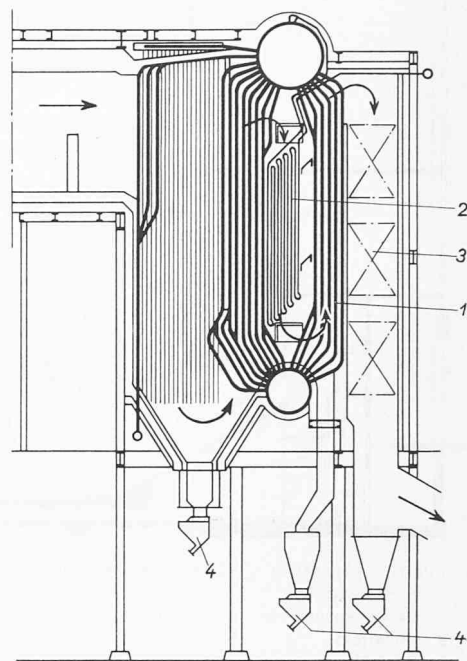
Bild 19. Abhitzekessel Hamburg
