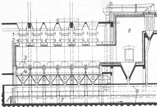
Bild 4. Längsschnitt durch einen Zellenofen. Bezeichnungen wie bei den Bildern 1 bis 3, dazu: 8 Verbrennungskammer, 9 Schlackenabfuhr
