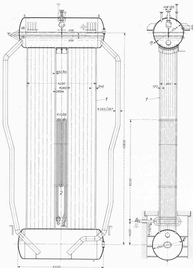
Bild 17. Abhitzekessel der Kehrichtverbrennungsanlage Lausanne, geliefert von der Schweiz, Lokomotiv- und Maschinenfabrik Winterthur 1 Verdampferrohre, 2 Ueberhitzerbündel
