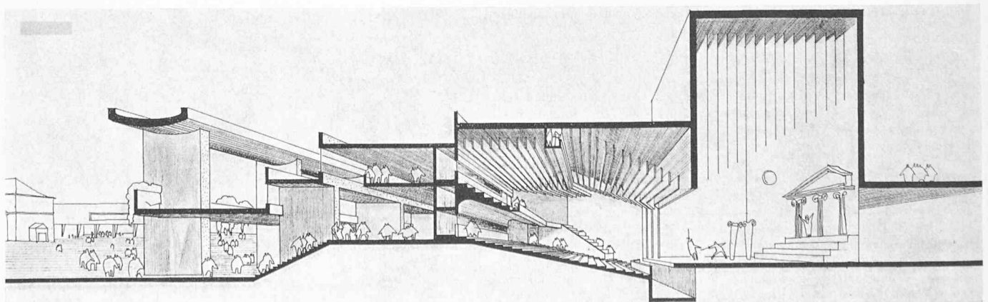
Perspektivischer Längsschnitt 1:900
