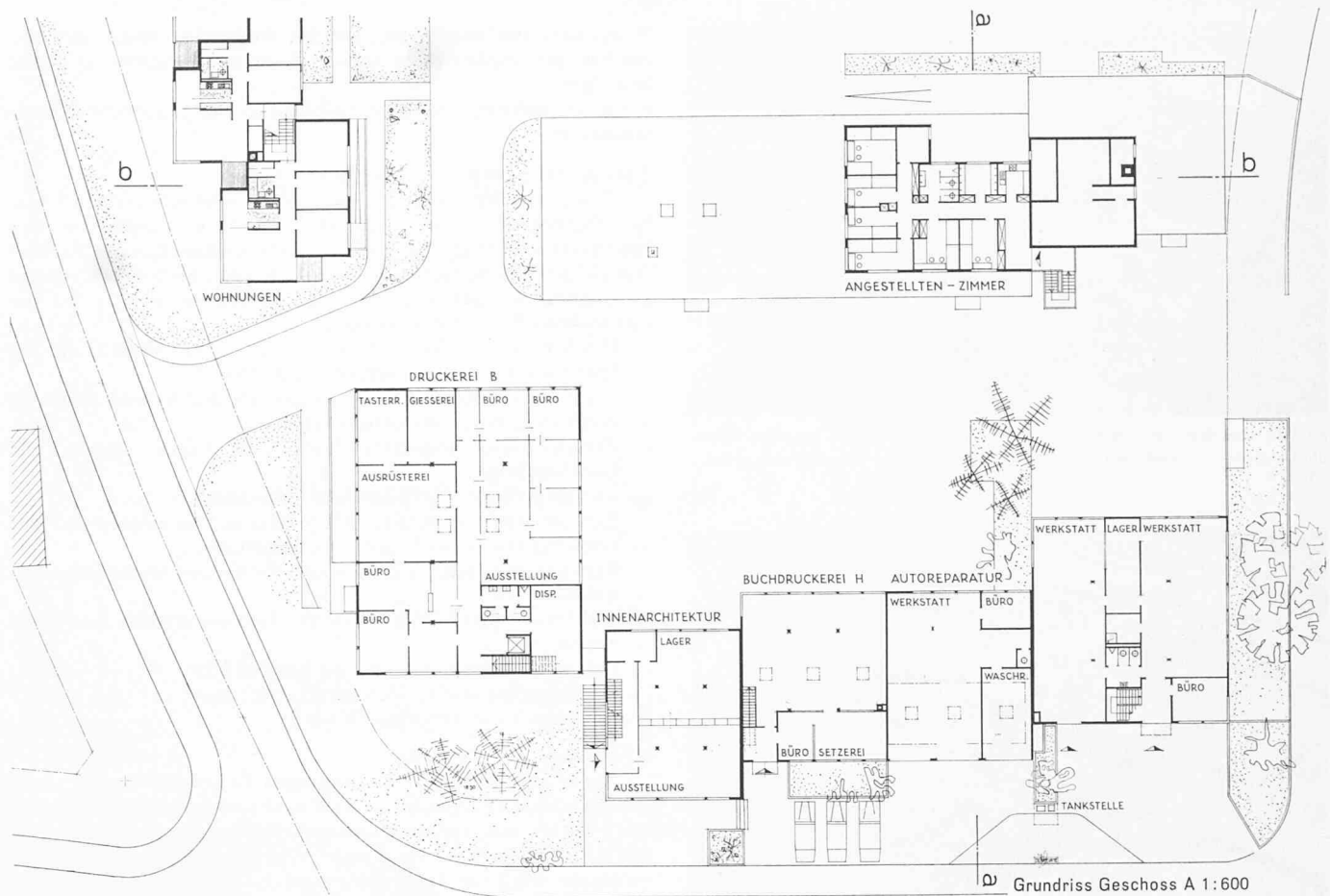
D Grundriss Geschoss A 1:600
