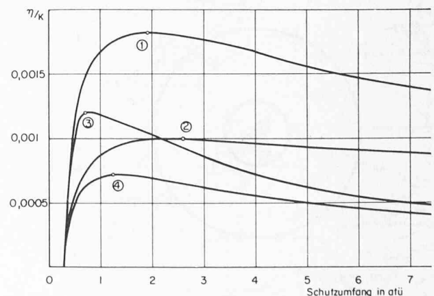
Bild 11. Resultat der Optimalisierung. Die besten Verhältnisse von Wirkungsgrad zu Schutzplatzkosten liegen im Bereich eines Schutzzumfanges von 0,75 bis 3 atü. Die Kurven beziehen sich auf die entsprechend bezeichneten Kostenrelationen von Bild 10
