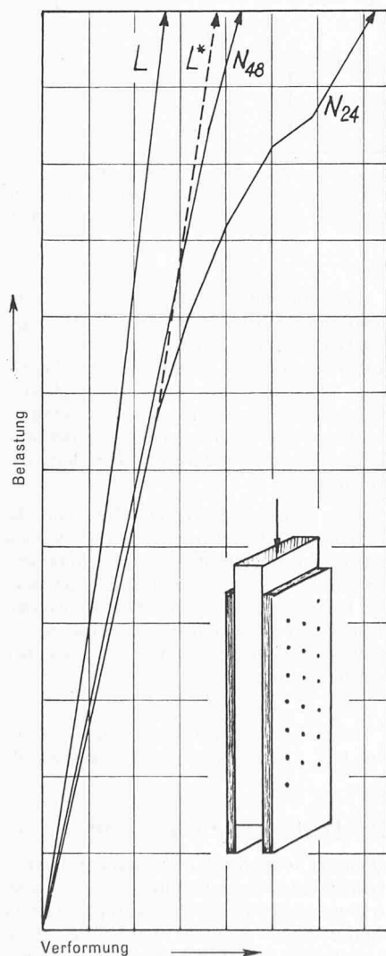
Bild 3. Last-Verformungsdiagramm von zweischschnittigen Druckscherkörpern mit Sperrholz-Laschen
