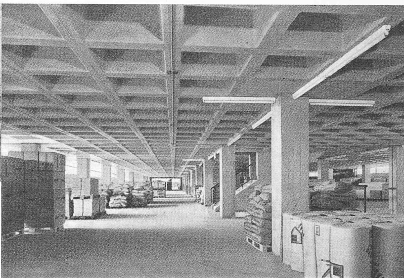
Bild 2 (rechts). Kassettendecke, deren Schalung aus Kunststoffcaissons gemäss Bild 1 hergestellt worden war
