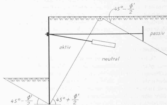
Bild 15. Verankerungszonen nach der klassischen Erddrucktheorie
