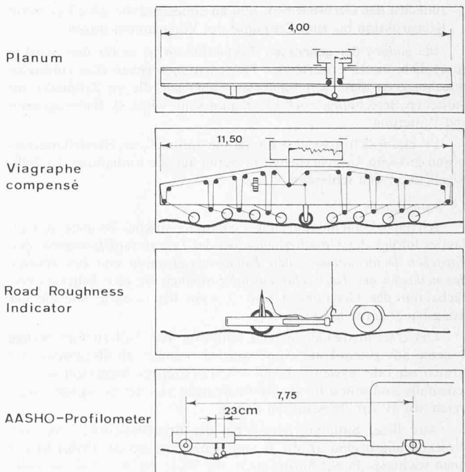
Bild 24. Ebenheitsmessgeräte
