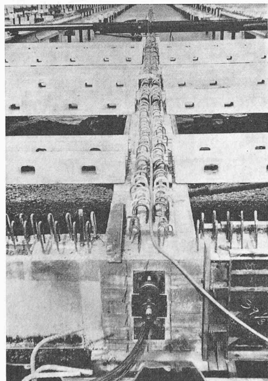
Bild 12 (links). Einziehen eines Kabels durch fünf aneinandergereihte vorfabrizierte L-Längsträger. Im Vordergrund Randträger in Ortsbeton. In Bildmitte Rippenplatten mit Aussparungen für Vorspannkabel, teilweise verlegt. Bügel für Anschluss des Plattenortsbetons
