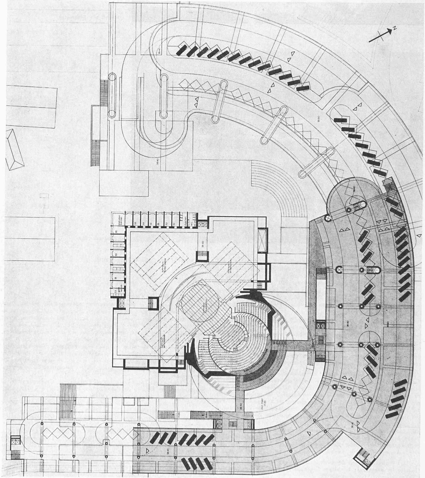
Hauptgeschoss 1:900
