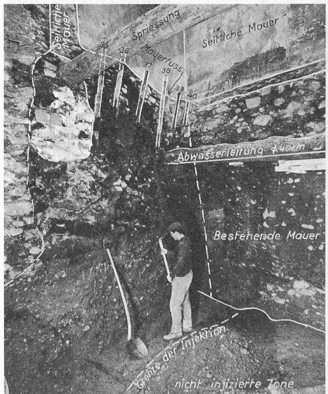
Bild 9. Baustelle in Genf. Aushub im injizierten Boden. 35 bis 40 = Manschettensrohre
