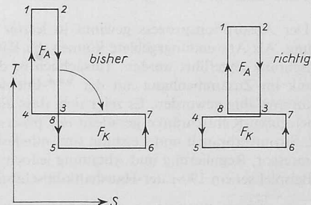
Bild 3. Bisherige und richtige T,s -Diagramme einstufiger Absorptionskältemaschinen
