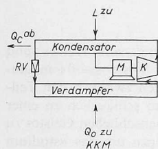
Bild 1a. Kreislaukschemata einer Kompressionskältemaschine (KKM) und einer Absorptionskältemaschine (AKM).
