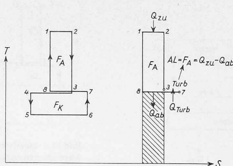
Bild 5. Idealisiertes T,s-Diagramm eines Kaltturbinen-Wärmeabfuhrsystems.
