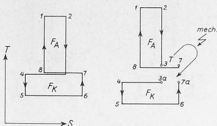
Bild 4. Idealisiertes T,s-Diagramm des Absorptionsprozesses. Dampfseitige Trennung in Antriebs- und Kälteabsorptionsprozess; äussere Kopplung durch mechanische oder elektrische Energie.
