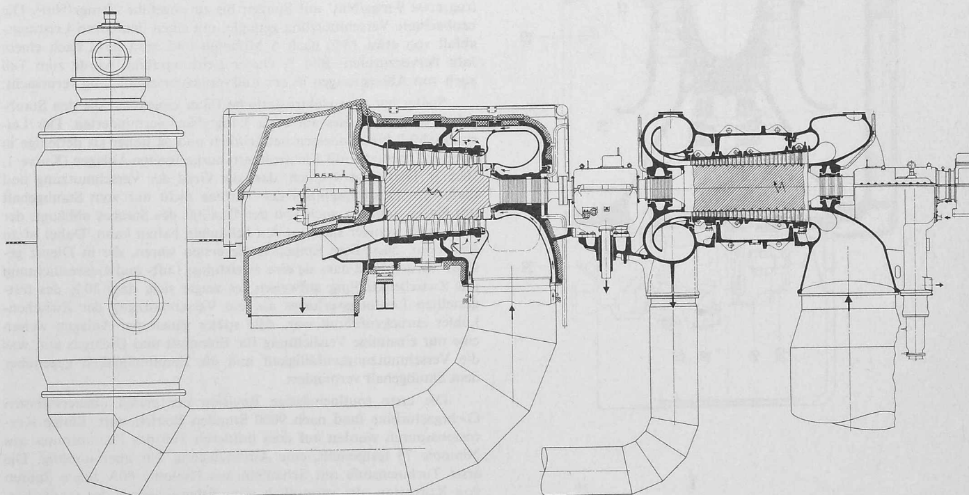
Bild 1. Längsschnitt durch eine Gasturbine grosser Leistung
