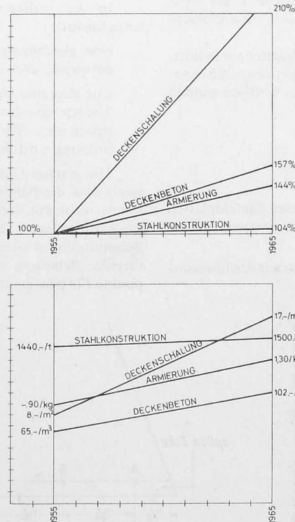
Bild 5. Vergleich der Kostenentwicklung Stahlkonstruktion-Ortbeton
