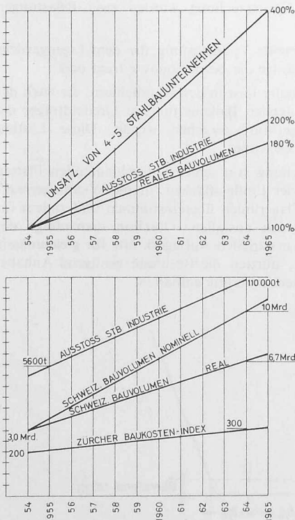
Bild 4. Bauvolumen und Ausstoss der schweizerischen Stahlbauindustrie
