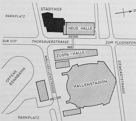
Lageplan 1:4500
