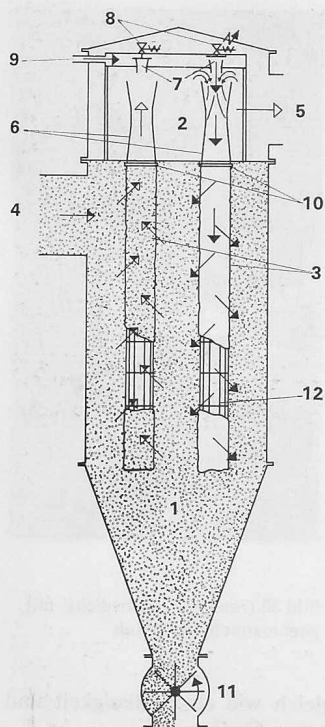
Bild 40. Düsenfilter mit Schlauchreinigung 1 Staubluftraum 2 Sauberluftkammer 3 Filterschläuche 4 Staubluft-Eintritt 5 Sauberluft-Austritt 6 Venturi-Rohr 7 Einblasdüsen 8 Ventile 9 Spüllufteintritt 10 Schnellschluss-Briden 11 Staubaustragschleuse 12 Drahtkörper zum Stützen der Schläuche 3
