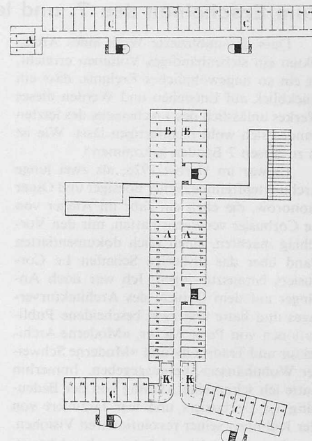
Plan d'un étage
