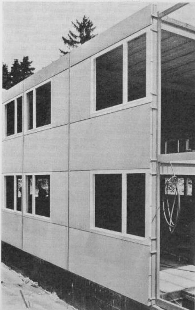
Aussenwand, 12 cm stark, mit Durisol-Fassadenplatten
