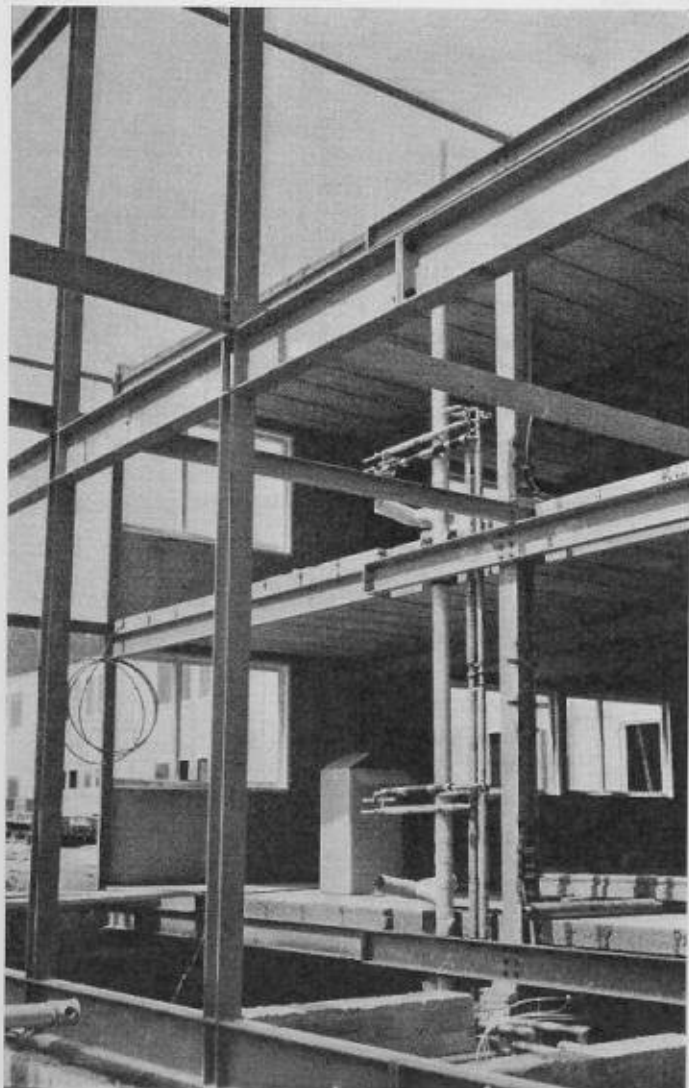
Stahlskelett mit Sanitärblock-Installation
