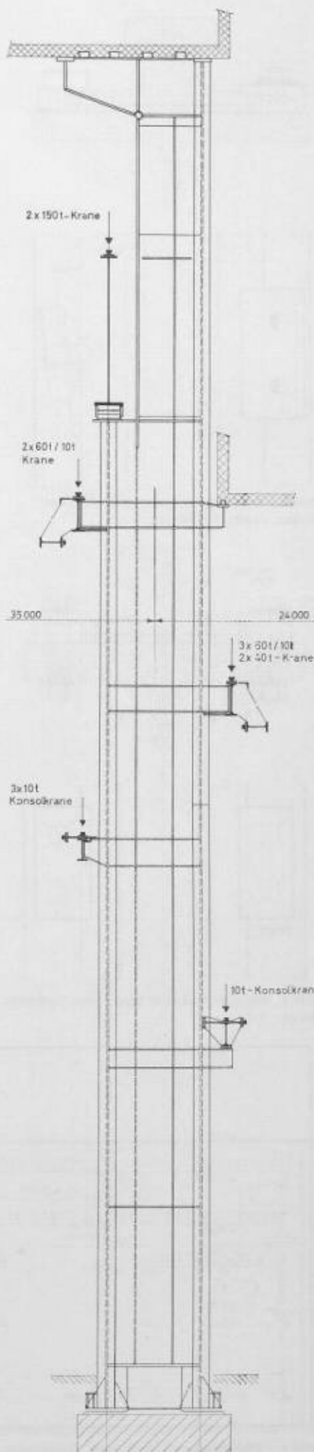
Bild 8. BBC-Neubauten im Birrfeld, Stütze in Axe 1090 mit Kranbahnen, 1:100
