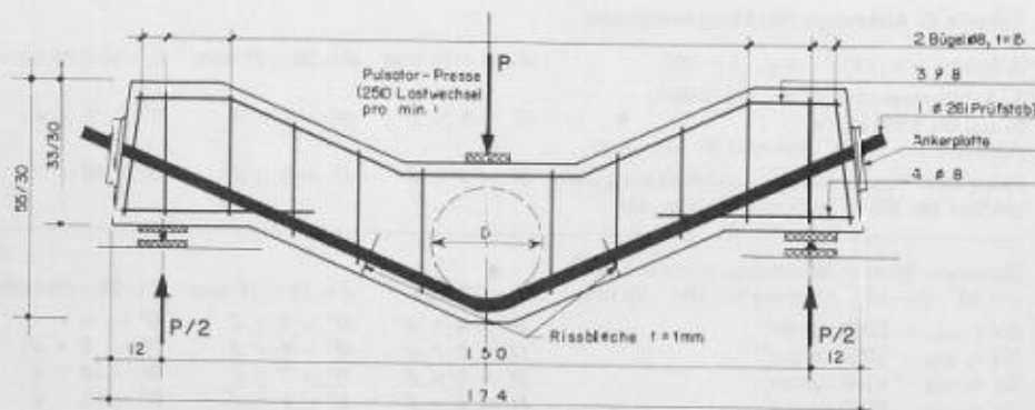
Bild 5. Versuchskörper zur Prüfung der Ermüdungsfestigkeit abgebogener Armierungsstähe [3]
