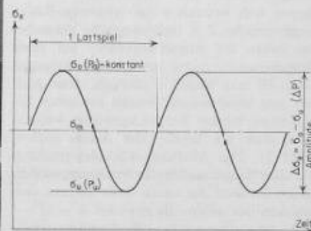
Bild 7. Zeit-Beanspruchungsdiagramm im Ermüdungsversuch
