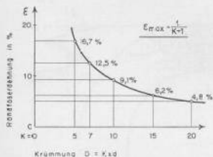
Bild 2. Dehnung der Randfasern und Eigenspannungen beim Kaltbiegen [2]
