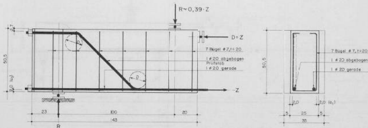
Bild 10. Anordnung älterer Versuche (1940) zur Prüfung abgelenkter Armierungen [4]
