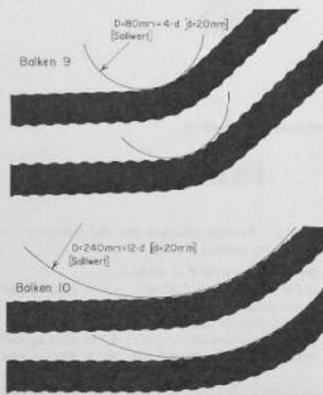
Bild 17. Abbiegungen von Stäben d = 20 mm (Box-Ultra)
