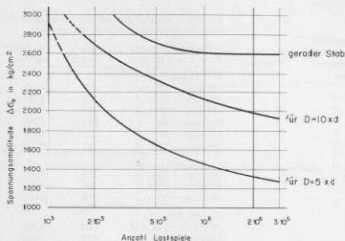
Bild 3. E-Müdigkeitsfestigkeit \Delta\sigma_e für gerade und abgelenkte Rippenstähle ( \sigma_s > 4000 \text{ kg/cm}^2 ) in Abhängigkeit von der Anzahl Lastwechsel (Wöhler-Diagramm)
