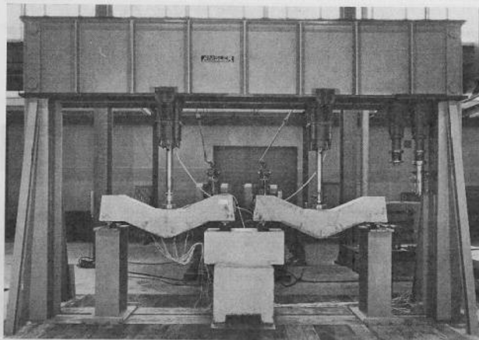
Bild 6. Versuchseinrichtung zur Prüfung der Ermüdungsfestigkeit abgebogener Armierungsstähe
