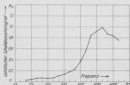
Bild 5. Statistischer Absorptionsgrad in Funktion der Frequenz von Stiflex-Belag direkt auf harter Unterlage
