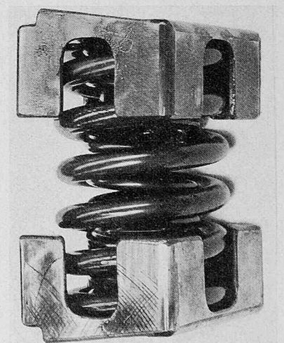
Bild 8. Federpaket
