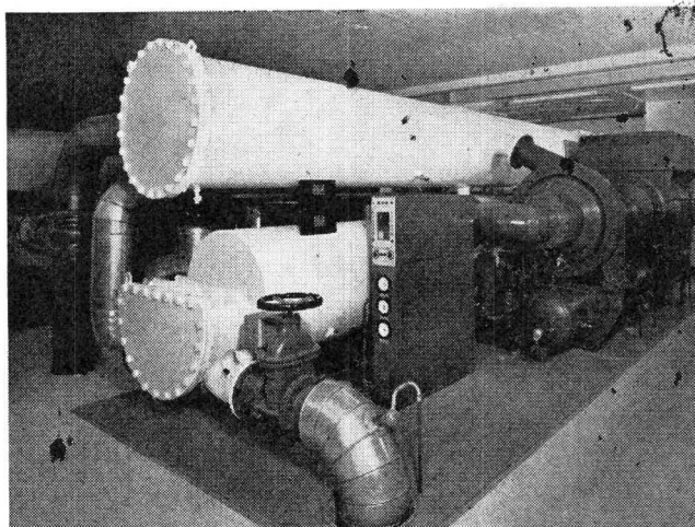
Sulzer-Uniturbo für Klimaanlage eines Bürohochhauses
