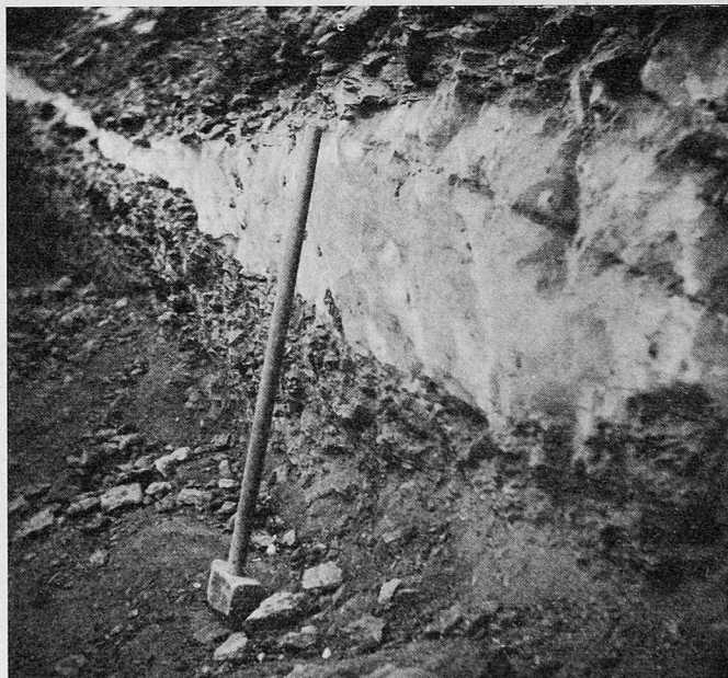
Bild 13. Permafrostlinie im Felsuntergrund der Gipfelstation
