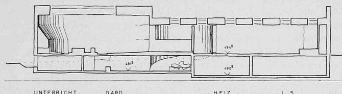
Schnitt B—B 1:600
