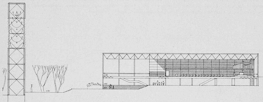
Schnitt A—A 1:600
