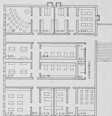
Zweites Untergeschoss 1:600 (vgl. Schnitt B—B)
