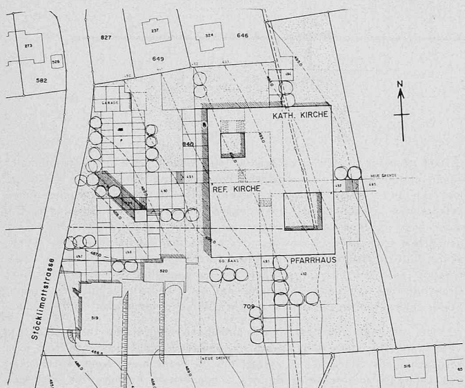
Lageplan 1:2000
