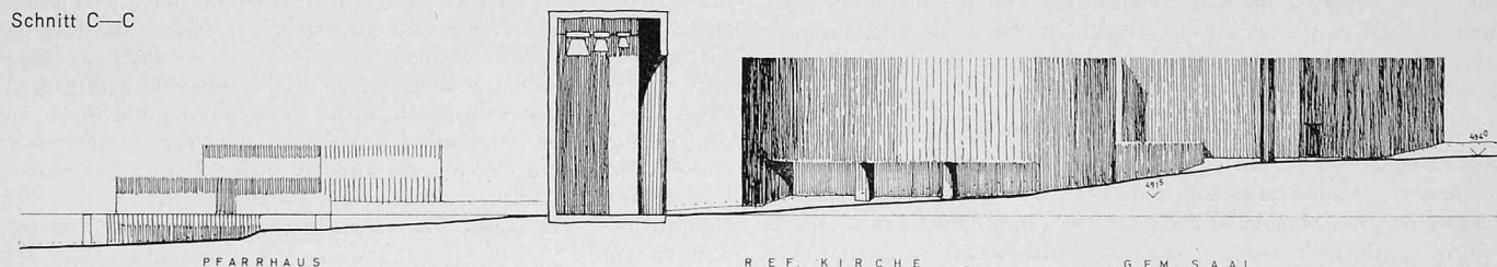
Schnitt C—C
