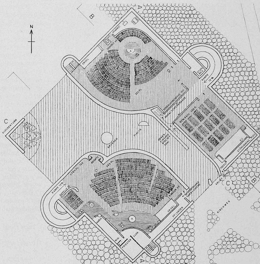
Hauptgeschoss 1:600
