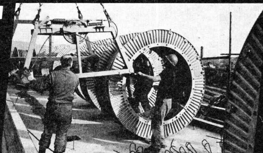
— Montage des Kranabrollgerätes
