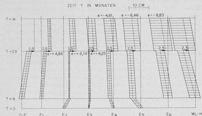
Bild 16. Brücke E: Pfeilerkopfbewegungen in Funktion der Zeit
