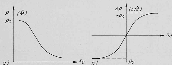
Bild 8. Kennlinien hydraulischer Transmitter bei der Erzeugung leistungsloser Signale
