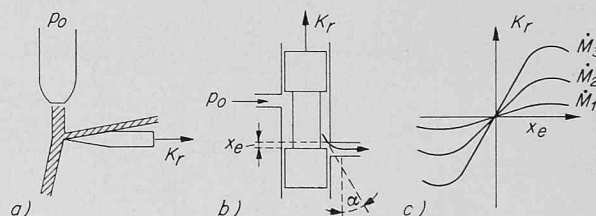
Bild 10. Strömungsmechanische Rückwirkungen in Signalerzeugungsorganen
