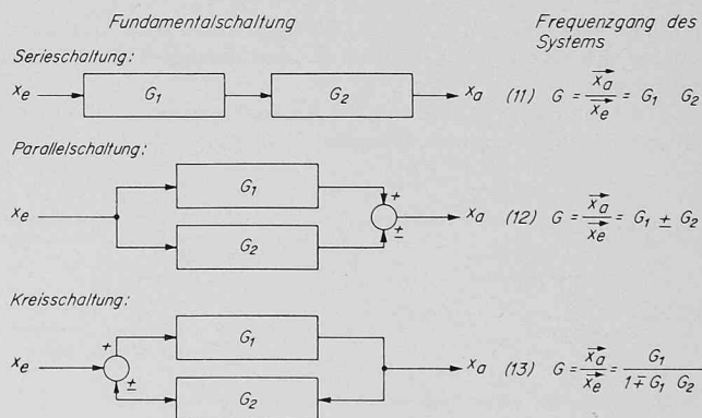
Bild 18. Berechnung des dynamischen Verhaltens von Systemen aus den dynamischen Eigenschaften ihrer Komponenten
