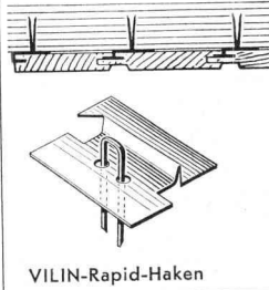
VILIN-Rapid-Haken
