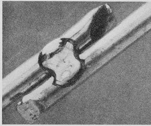
Bild 9a. Punktschweißen zweier Drähte aus Ni mit 0,5 mm Durchmesser [20]
