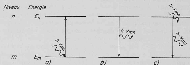
Bild 1. Die drei möglichen Arten von Uebergängen eines Atoms in einem atomischen System
