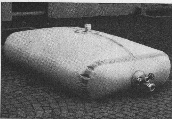
Bild 1. Geschlossener EXCALOR-Falttank aus Perbunan-beschichtetem Polyestergewebe (Trevira) für Wasser, Öl oder Chemikalien; Fassungsvermögen 1000 l.
