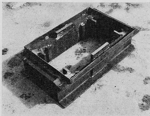
Bild 6. Stahlkragen
